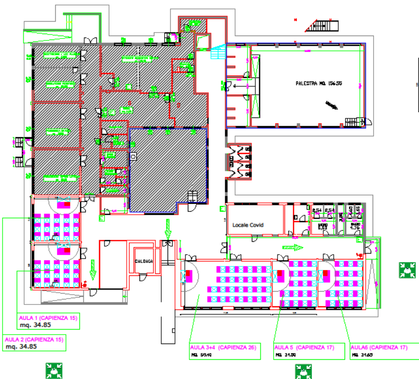
PIANTA PIANO TERRA - Primaria
